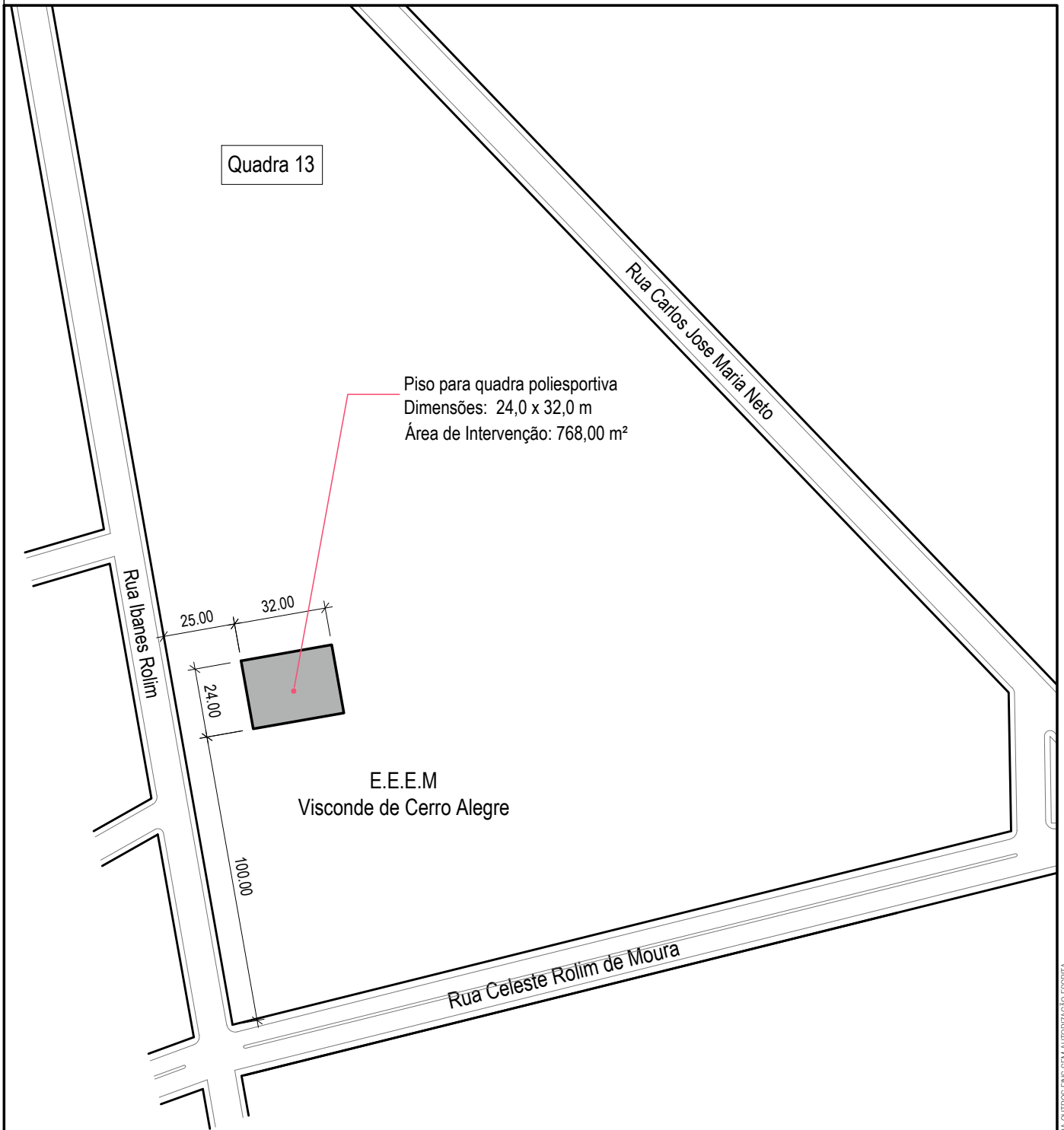
01 PLANTA DE SITUAÇÃO / LOCALIZAÇÃO Escala 1:2.000
